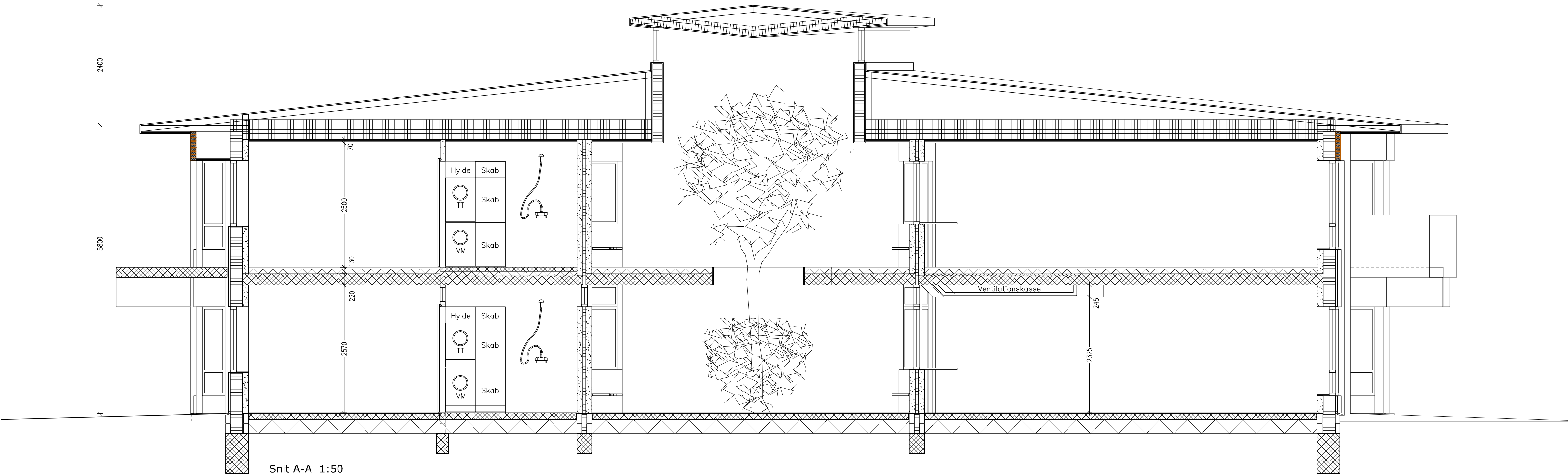
Snit A-A 1:50
